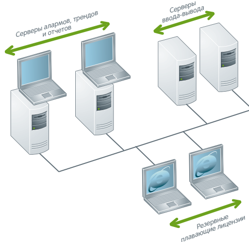
Архитектура с резервированием, отдельные серверы АТО и ввода-вывода, с 2 лицензиями оператора и 2 веб-лицензиями руководителя
